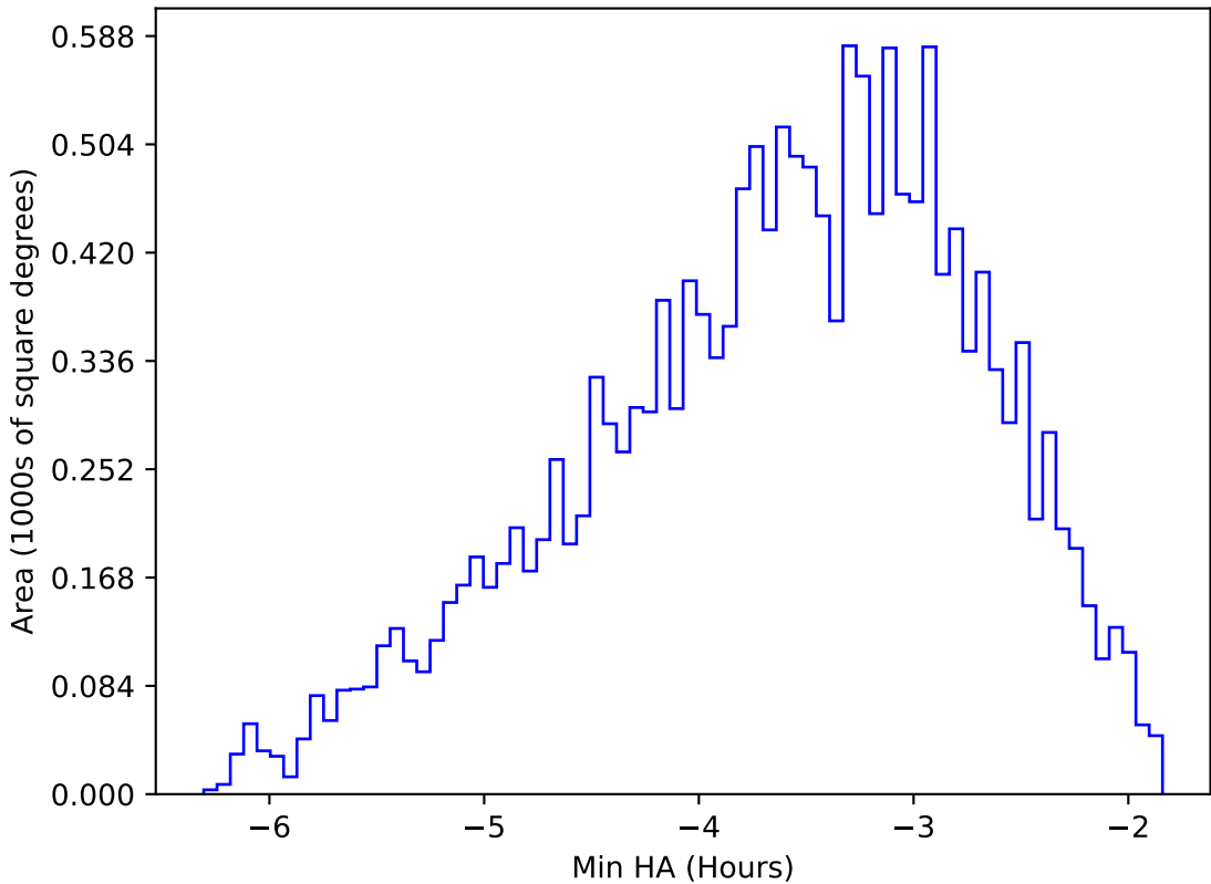
too_elab_heavy_r64_d2_ugrizy_v3.4_10yrs WFD y band: Min HA
