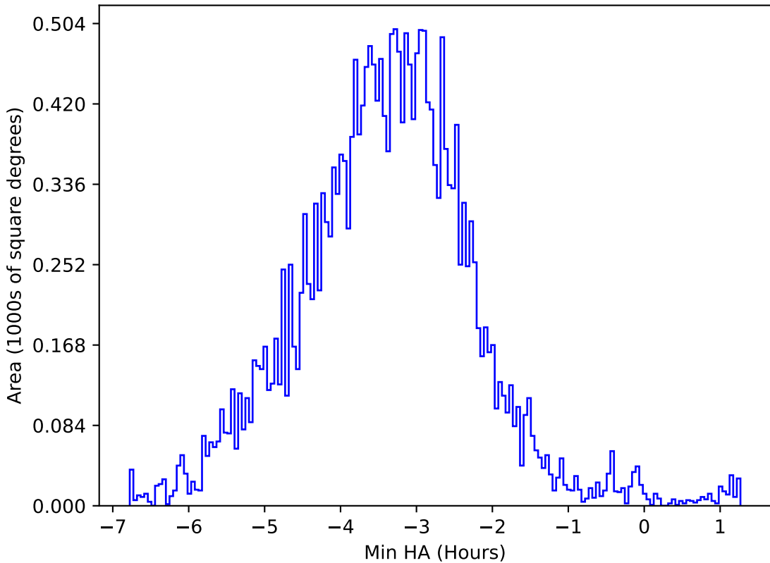
too_elab_heavy_r64_d2_ugrizy_v3.4_10yrs All sky y band: Min HA
