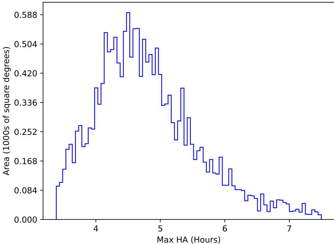
too_elab_heavy_r64_d2_ugrizy_v3.4_10yrs WFD y band: Max HA
