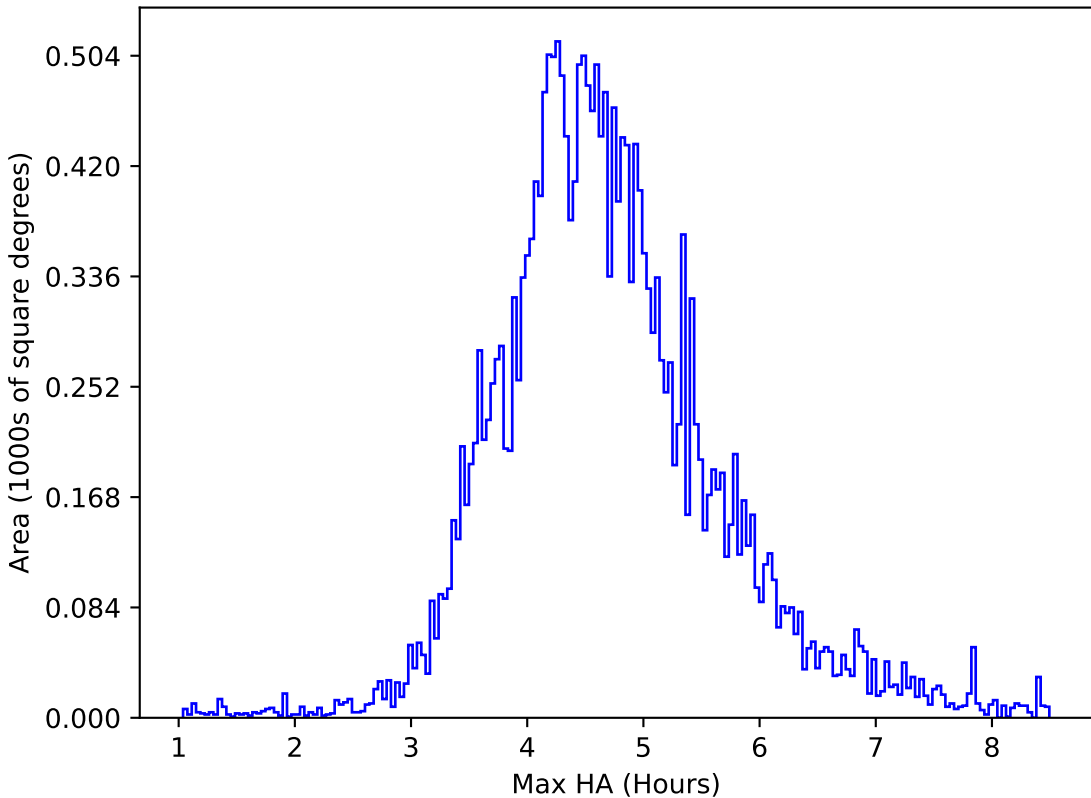
too_elab_heavy_r64_d2_ugrizy_v3.4_10yrs All sky y band: Max HA
