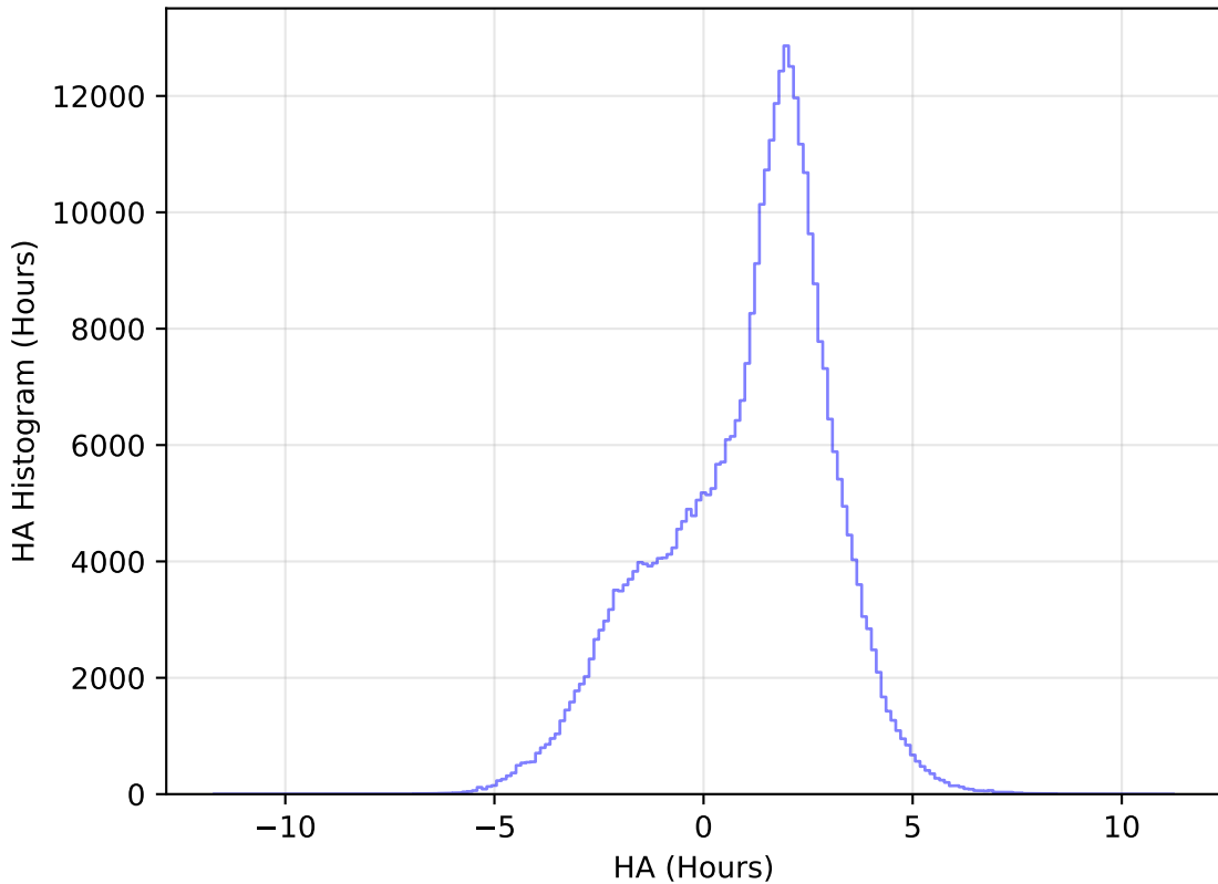
too_elab_heavy_r64_d2_ugrizy_v3.4_10yrs WFD y band: HA Histogram
