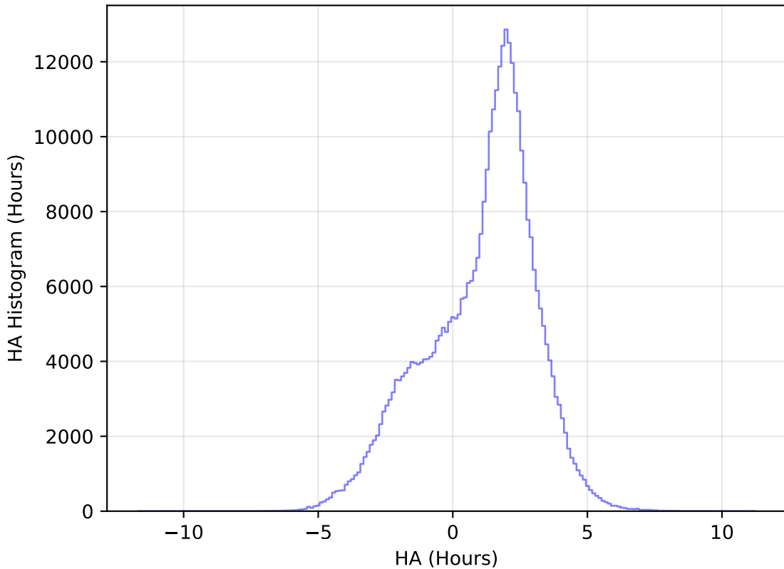
too_elab_heavy_r64_d2_ugrizy_v3.4_10yrs All sky y band: HA Histogram
