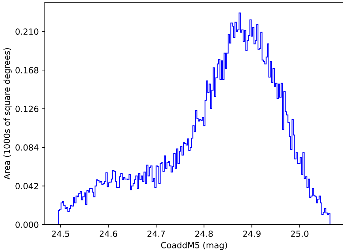
too_elab_heavy_r64_d2_ugrizy_v3.4_10yrs WFD y band: CoaddM5
