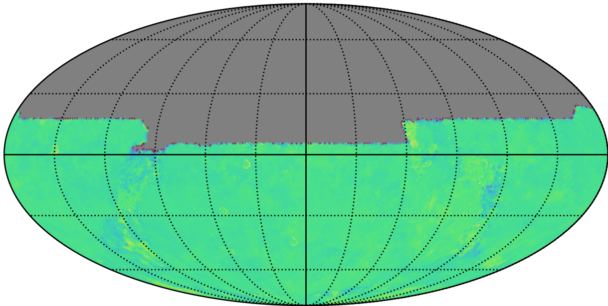
too_elab_heavy_r64_d2_gz_v3.4_10yrs u: Kuiper rotTelPos
