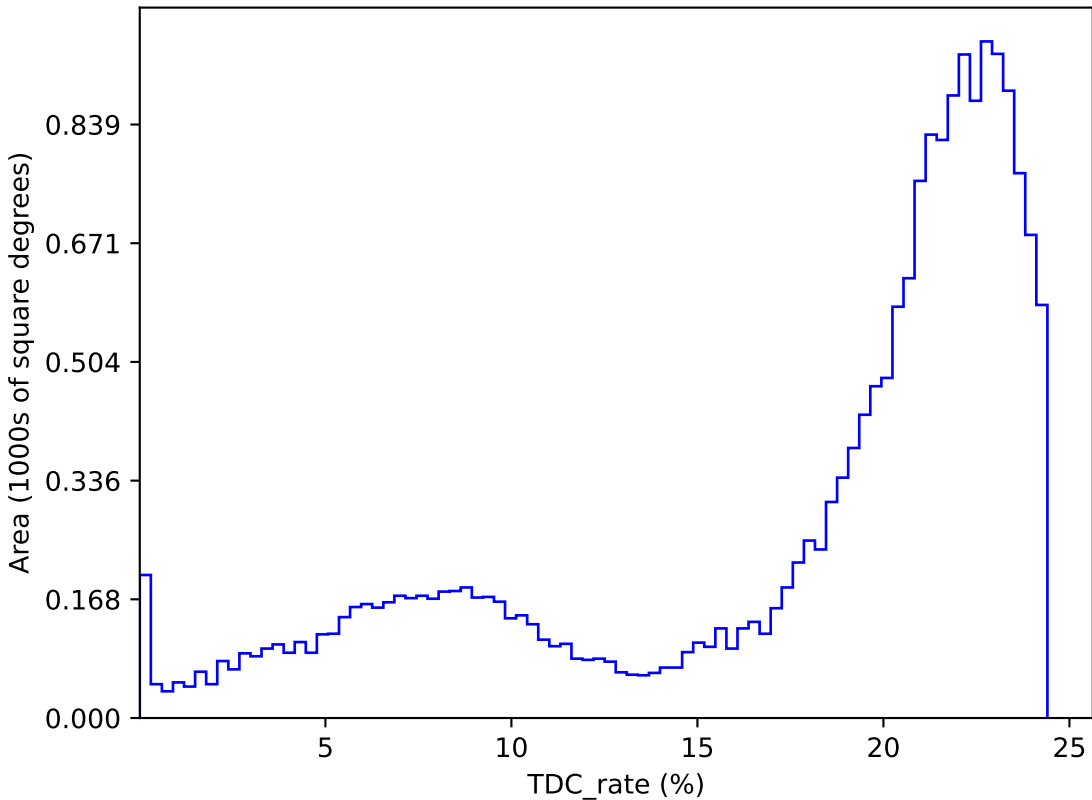
too_elab_heavy_r32_d3_ugrizy_v3.4_10yrs : TDC_rate
