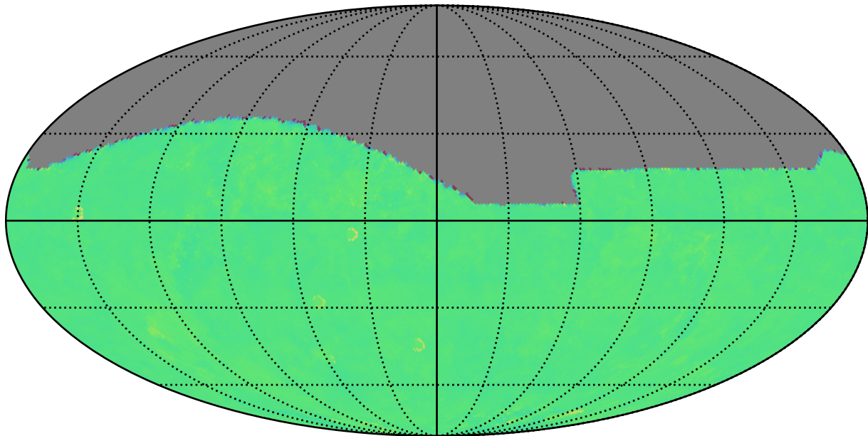
too_elab_heavy_r32_d3_ugrizy_v3.4_10yrs i: Kuiper rotTelPos
