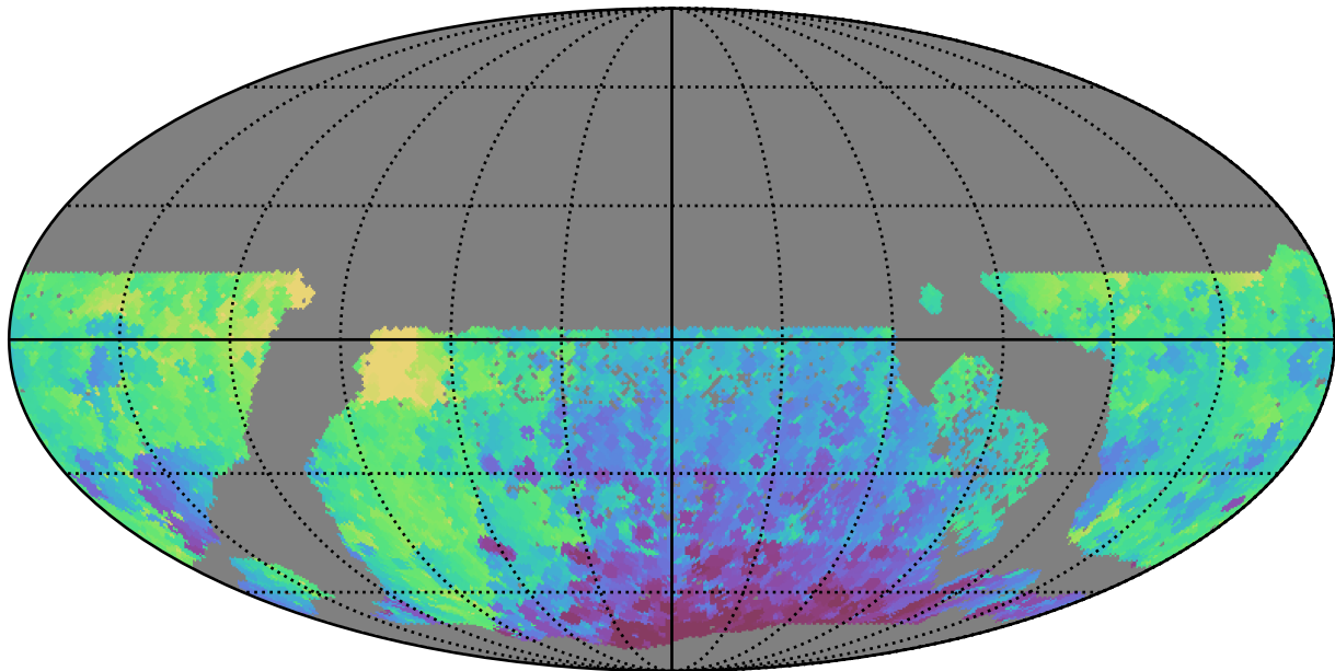
too_elab_heavy_r32_d3_ugrizy_v3.4_10yrs WFD y band: Min HA
