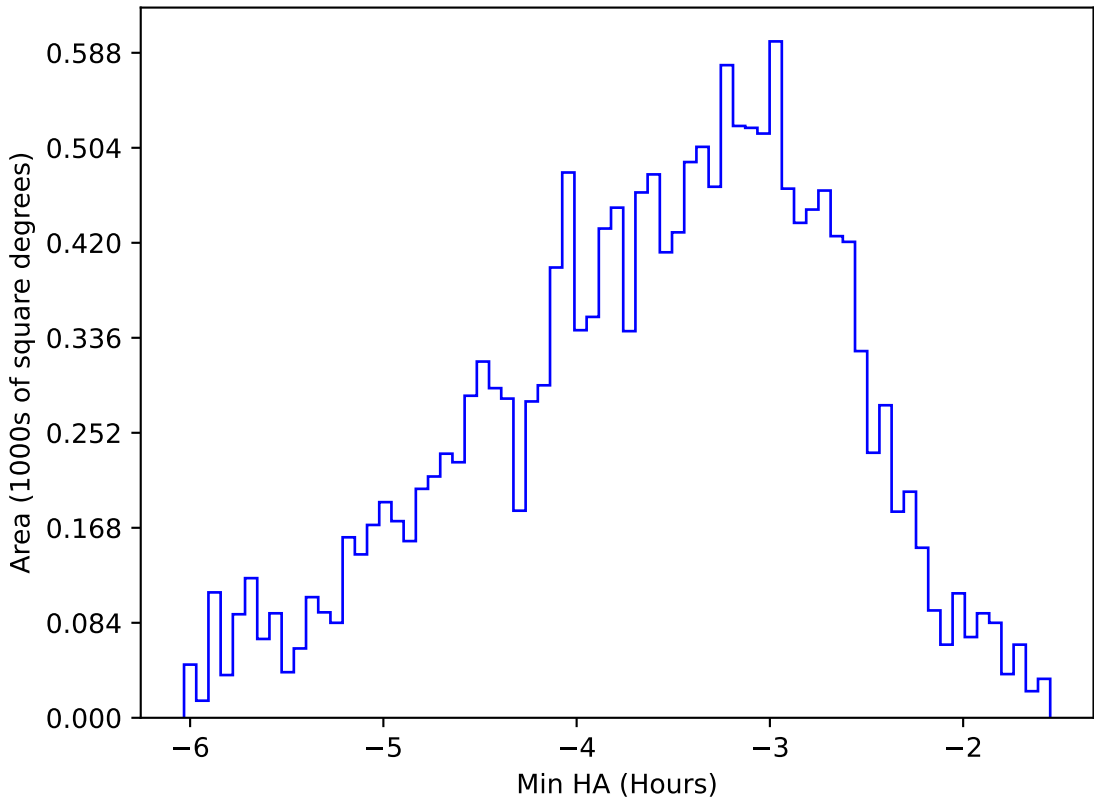
too_elab_heavy_r32_d3_ugrizy_v3.4_10yrs WFD y band: Min HA
