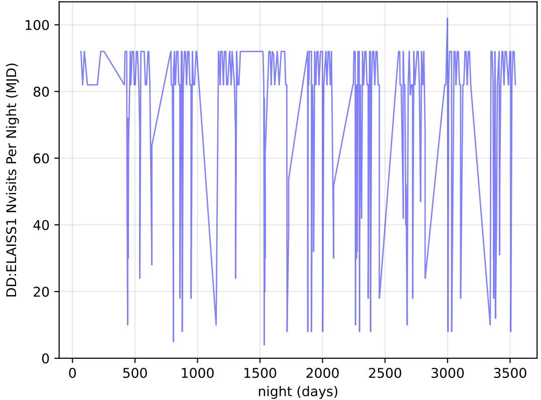
too_elab_heavy_r32_d3_ugrizy_v3.4_10yrs all bands: DD:ELAISS1 Nvisits Per Night
