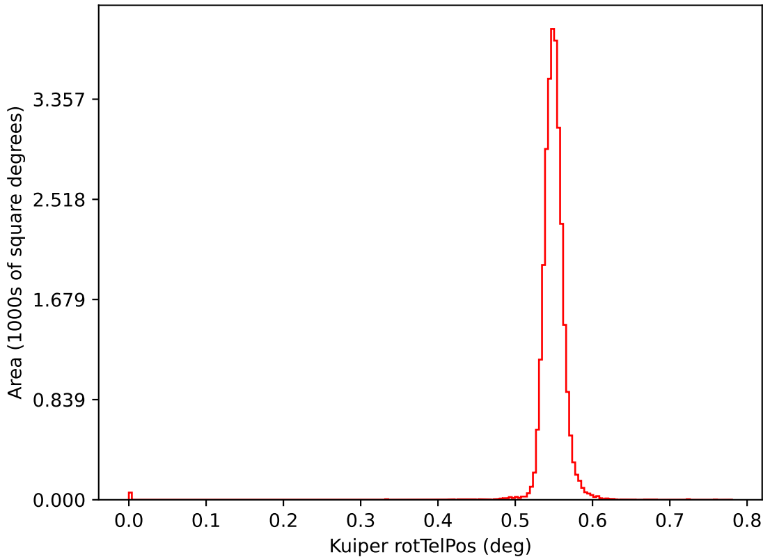
too_elab_heavy_r32_d3_gz_v3.4_10yrs i: Kuiper rotTelPos
