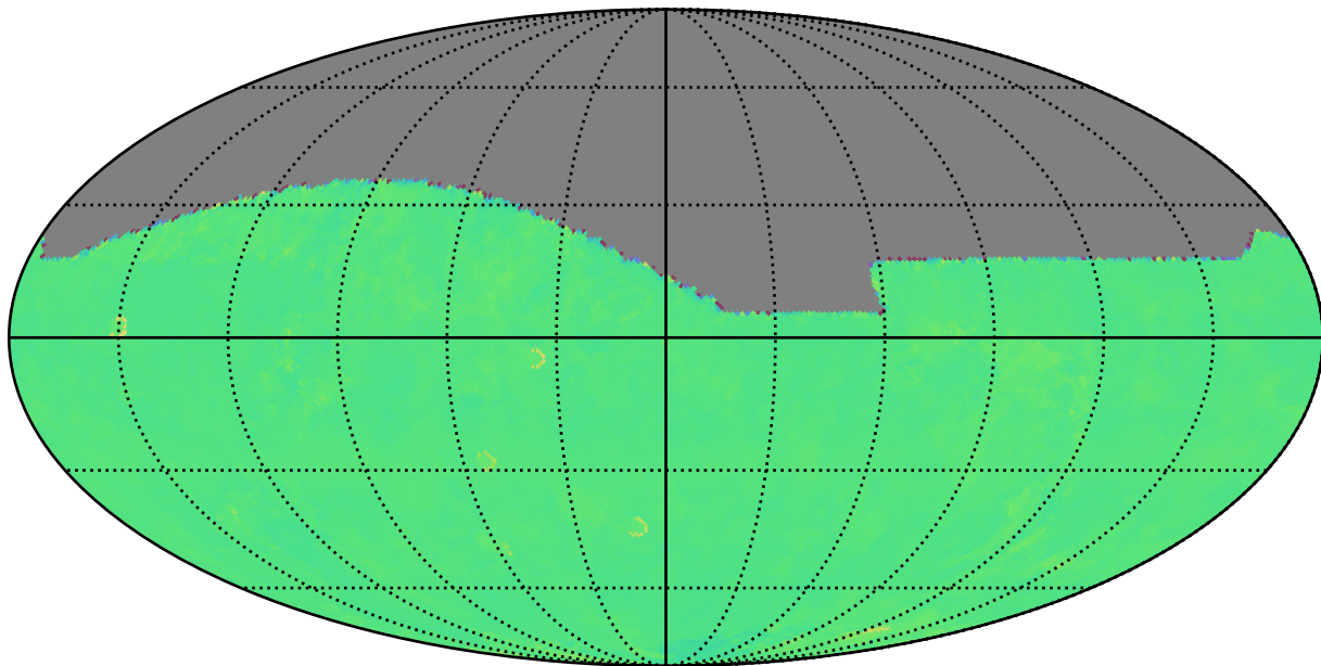
too_elab_heavy_r32_d3_griz_v3.4_10yrs i: Kuiper rotTelPos
