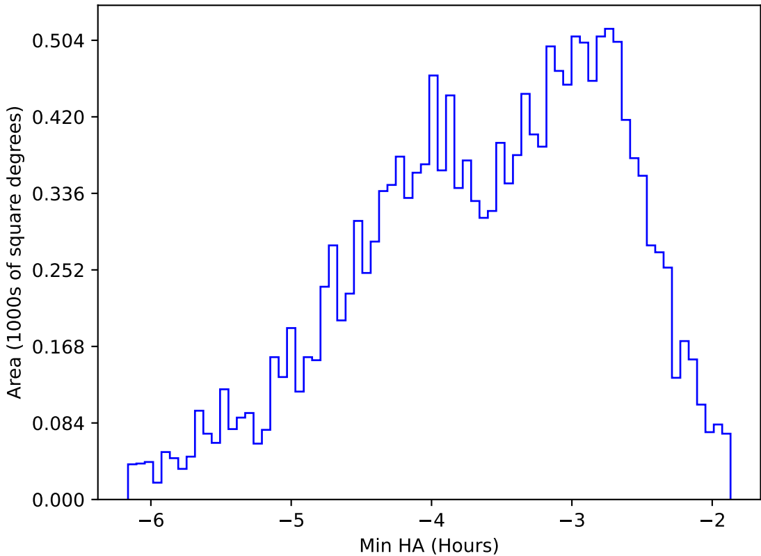
too_elab_heavy_r32_d2_ugrizy_v3.4_10yrs WFD y band: Min HA
