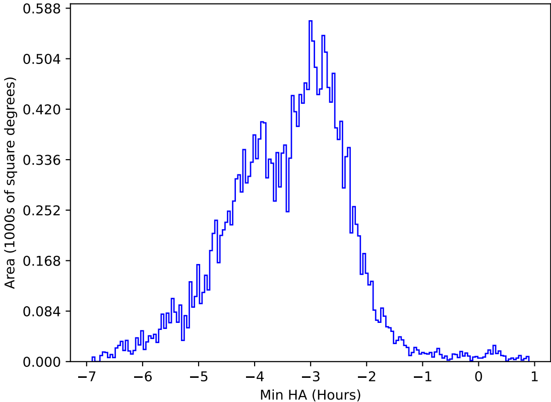
too_elab_heavy_r32_d2_ugrizy_v3.4_10yrs All sky y band: Min HA
