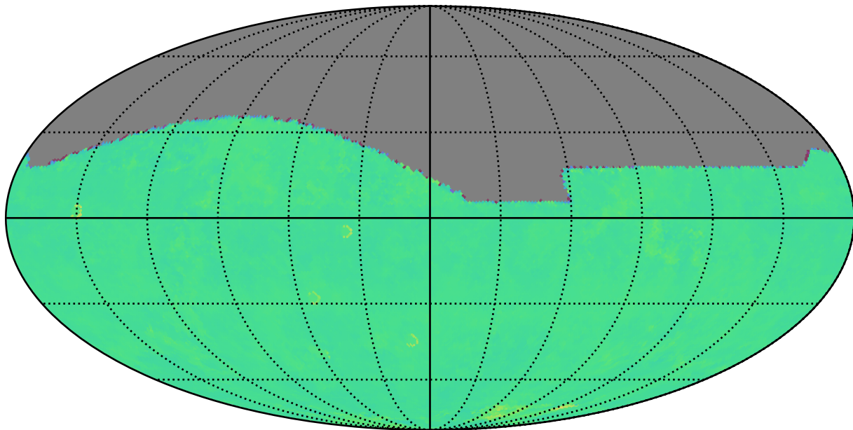
too_elab_heavy_r32_d2_griz_v3.4_10yrs i: Kuiper rotTelPos
