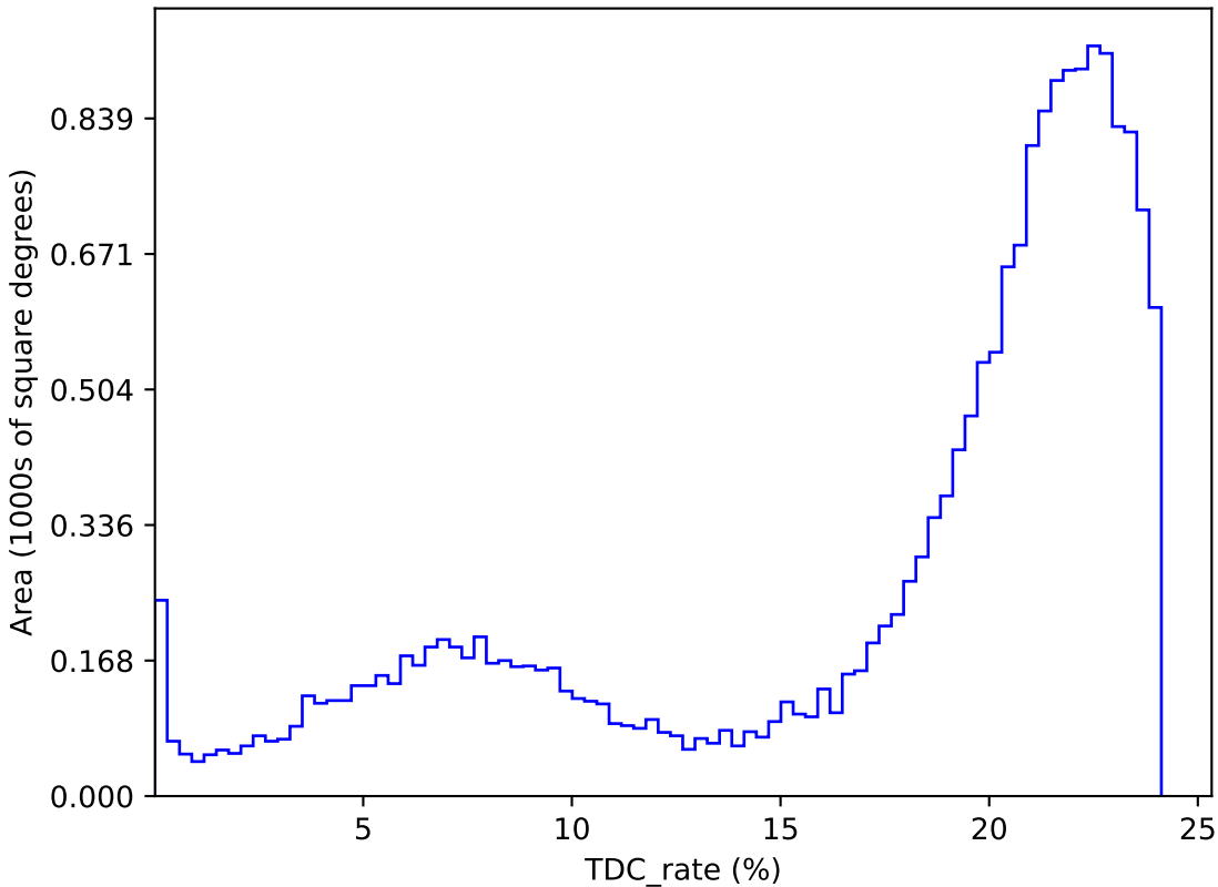
too_elab_heavy_r128_d3_ugrizy_v3.4_10yrs : TDC_rate
