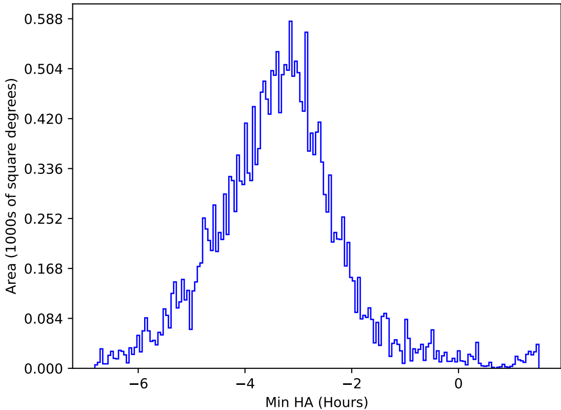
too_elab_heavy_r128_d3_ugrizy_v3.4_10yrs All sky y band: Min HA
