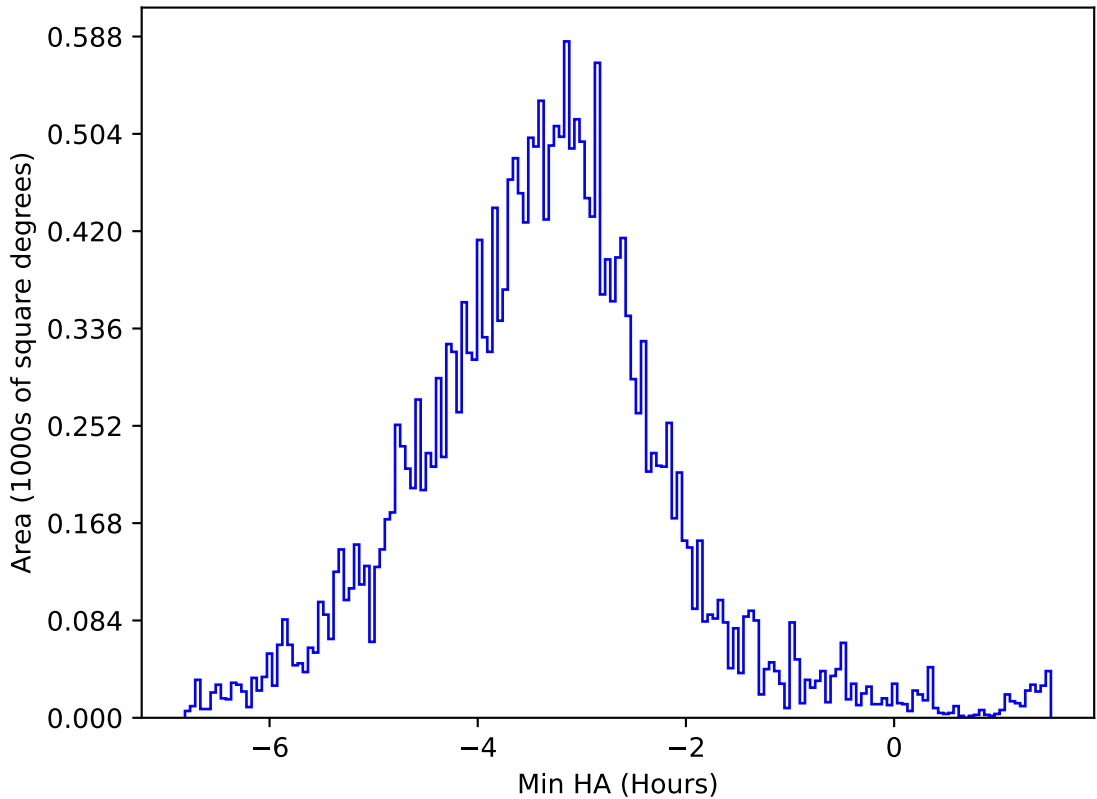
too_elab_heavy_r128_d3_ugrizy_v3.4_10yrs All sky y band: Min HA
