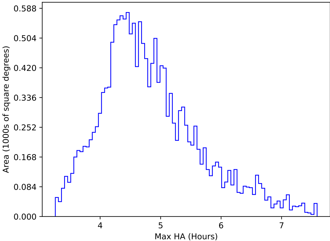
too_elab_heavy_r128_d3_ugrizy_v3.4_10yrs WFD y band: Max HA
