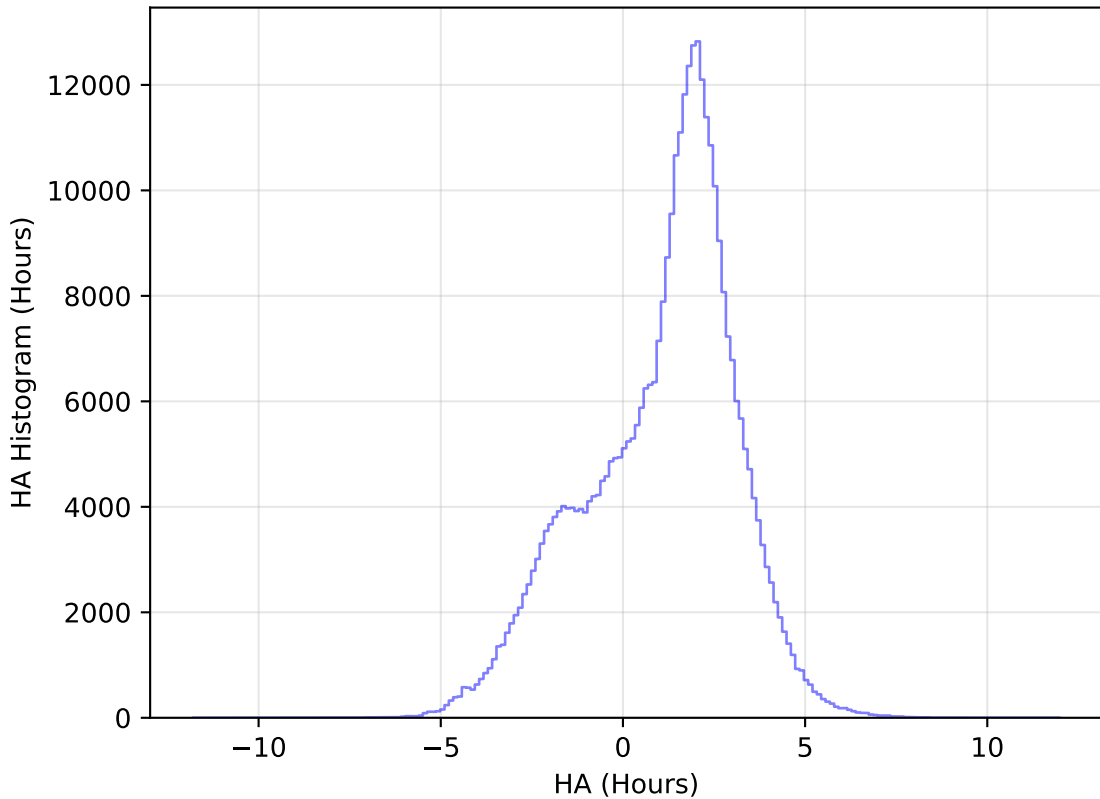
too_elab_heavy_r128_d3_ugrizy_v3.4_10yrs All sky y band: HA Histogram
