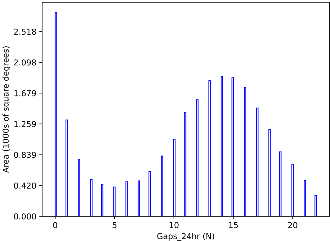
too_elab_heavy_r128_d2_ugrizy_v3.4_10yrs y band: Gaps_24hr
