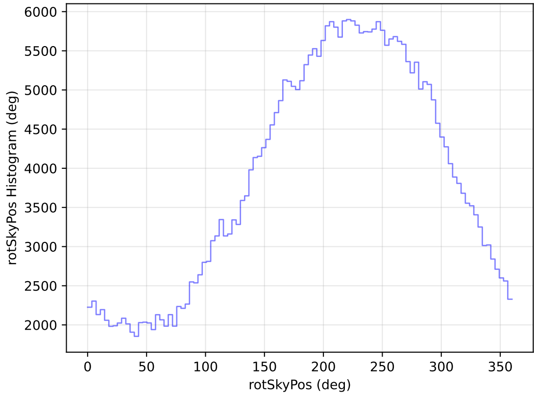
too_elab_heavy_r128_d2_ugrizy_v3.4_10yrs All sky y band: rotSkyPos Histogram
