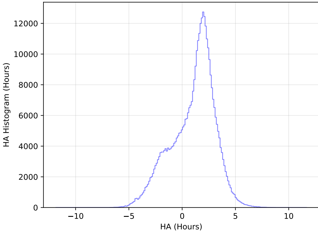
too_elab_heavy_r128_d2_ugrizy_v3.4_10yrs WFD y band: HA Histogram
