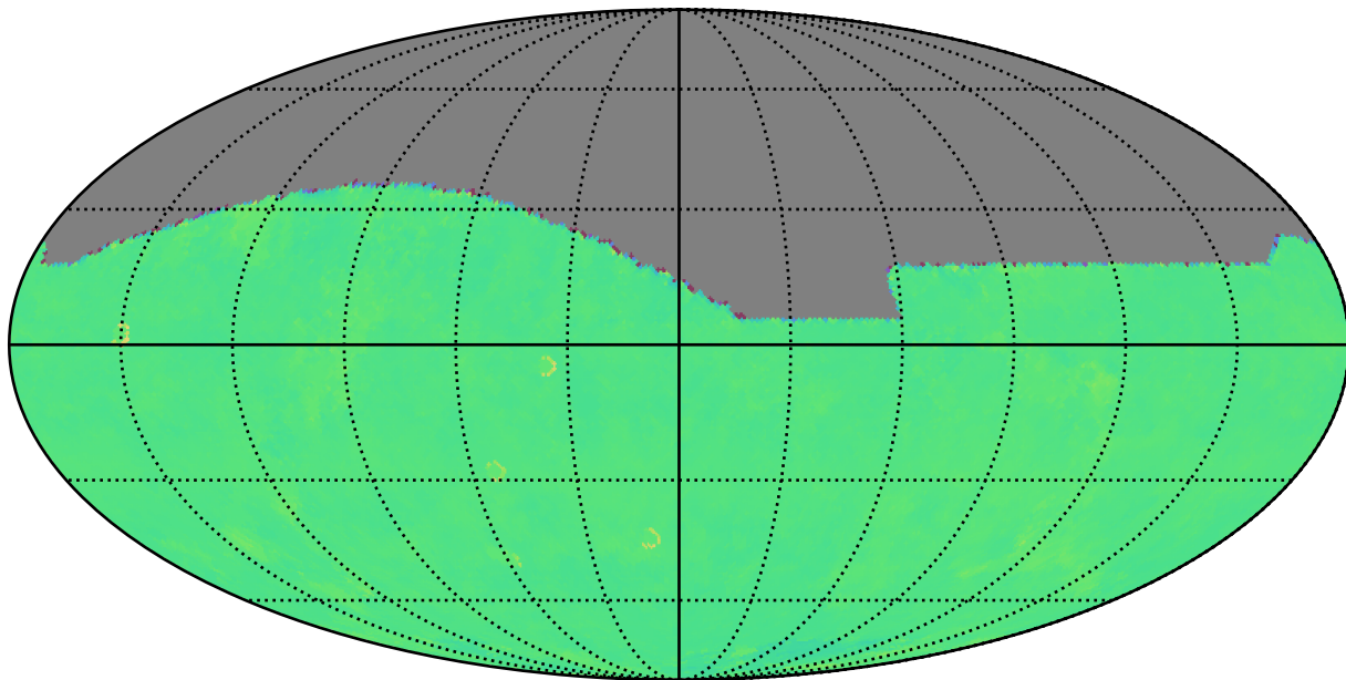
too_elab_heavy_r128_d2_gz_v3.4_10yrs i: Kuiper rotTelPos
