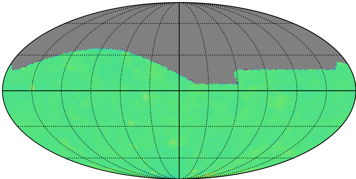
too_elab_2yr_r64_d3_ugrizy_v3.4_10yrs r: Kuiper rotTelPos
