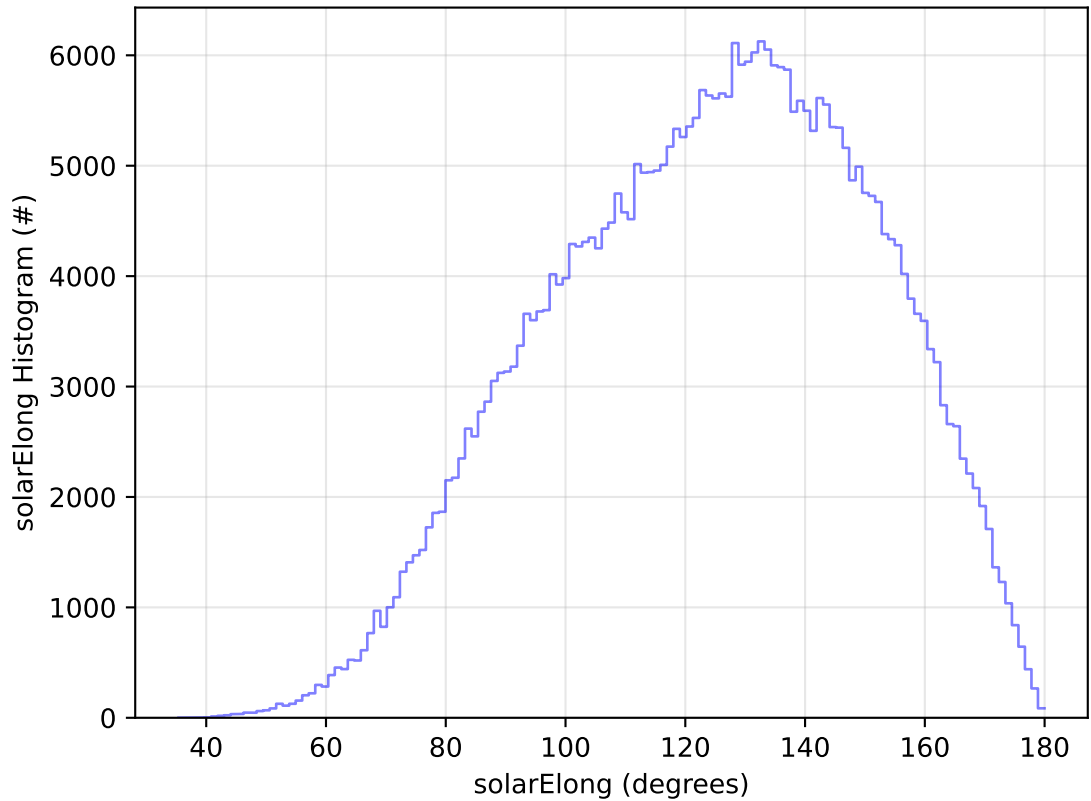
too_elab_2yr_r64_d3_ugrizy_v3.4_10yrs WFD y band: solarElong Histogram
