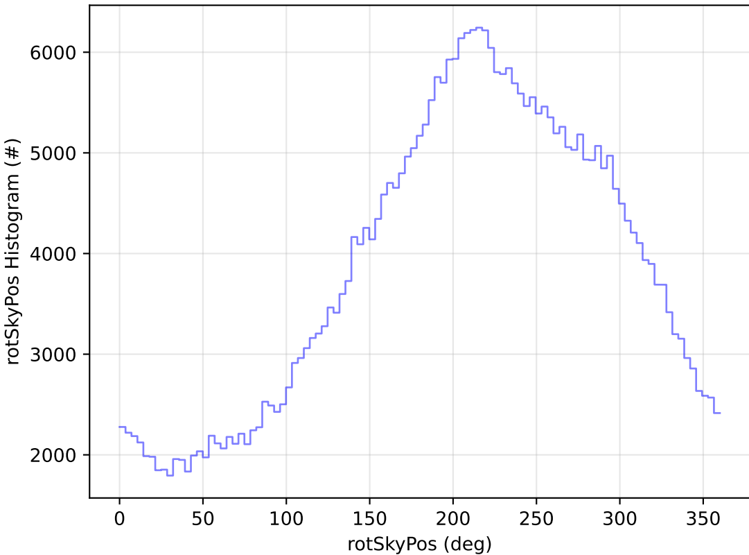
too_elab_2yr_r64_d3_ugrizy_v3.4_10yrs WFD y band: rotSkyPos Histogram
