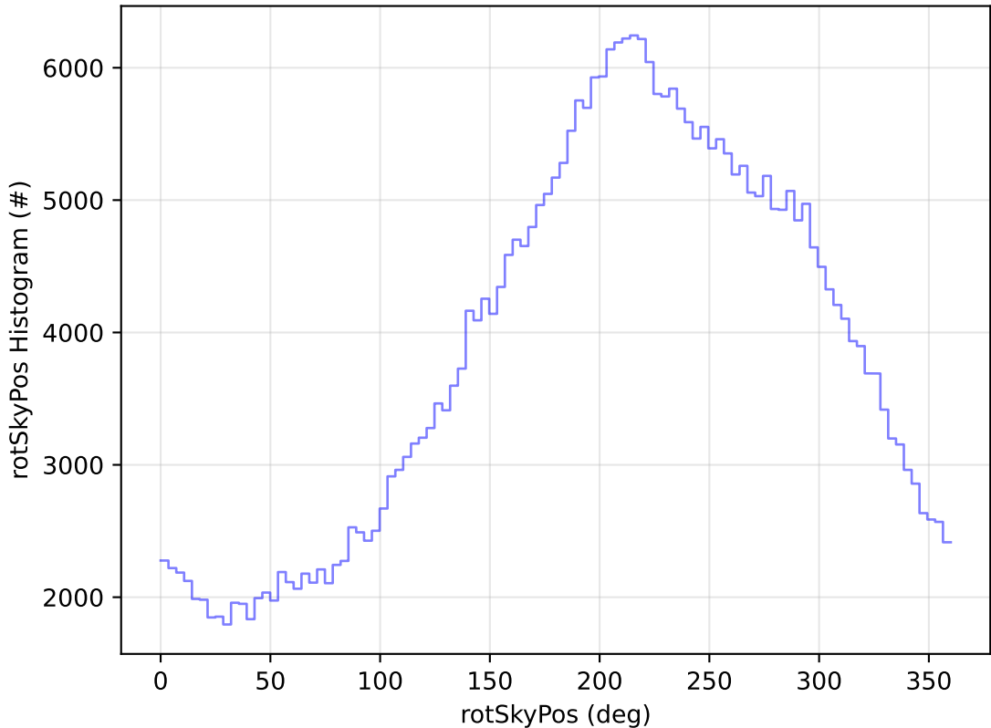
too_elab_2yr_r64_d3_ugrizy_v3.4_10yrs All sky y band: rotSkyPos Histogram
