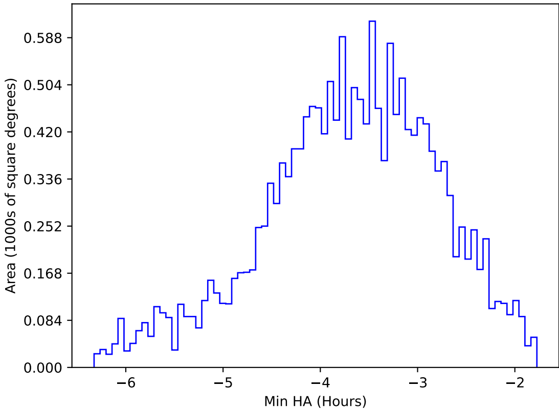
too_elab_2yr_r64_d3_ugrizy_v3.4_10yrs WFD y band: Min HA
