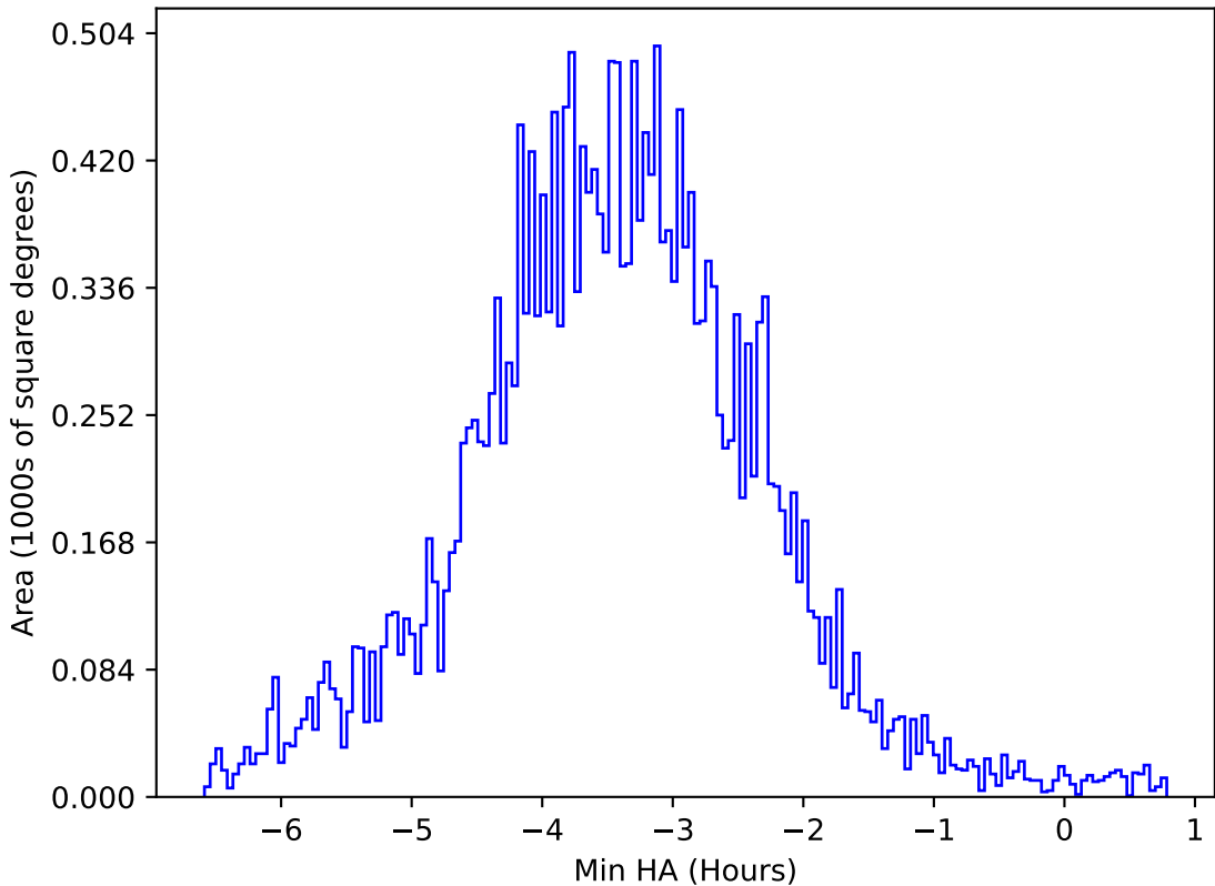
too_elab_2yr_r64_d3_ugrizy_v3.4_10yrs All sky y band: Min HA
