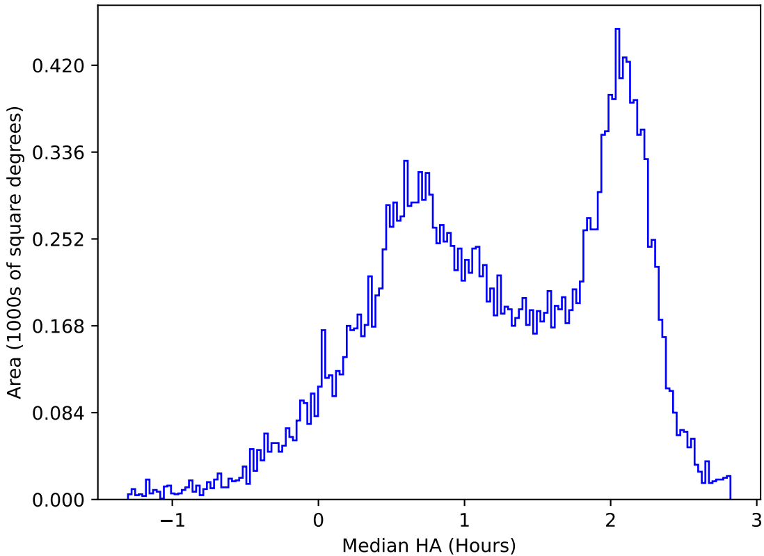
too_elab_2yr_r64_d3_ugrizy_v3.4_10yrs All sky y band: Median HA
