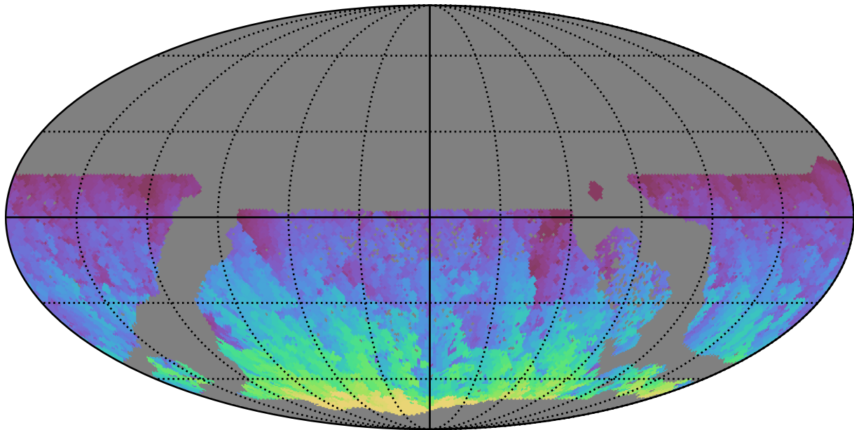
too_elab_2yr_r64_d3_ugrizy_v3.4_10yrs WFD y band: Max HA
