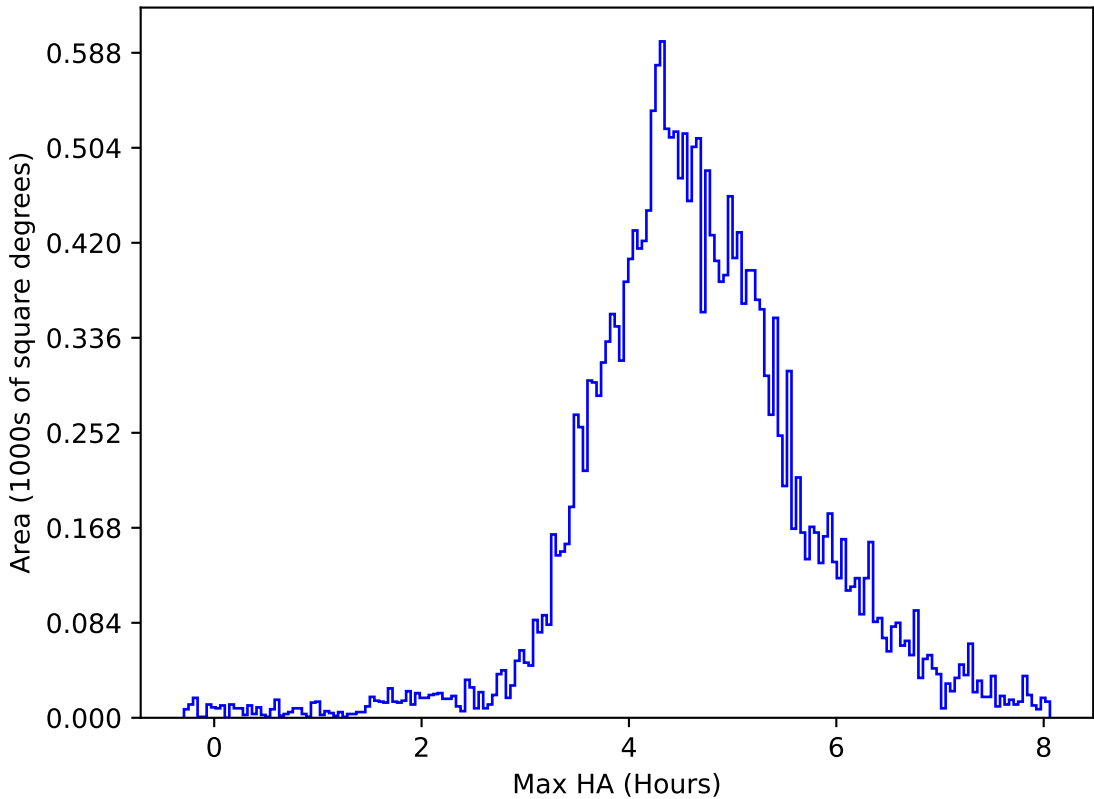
too_elab_2yr_r64_d3_ugrizy_v3.4_10yrs All sky y band: Max HA
