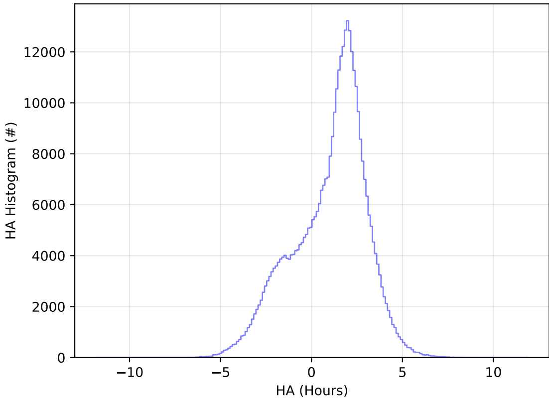
too_elab_2yr_r64_d3_ugrizy_v3.4_10yrs WFD y band: HA Histogram
