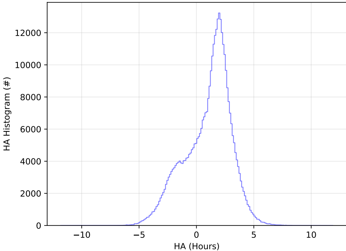
too_elab_2yr_r64_d3_ugrizy_v3.4_10yrs All sky y band: HA Histogram
