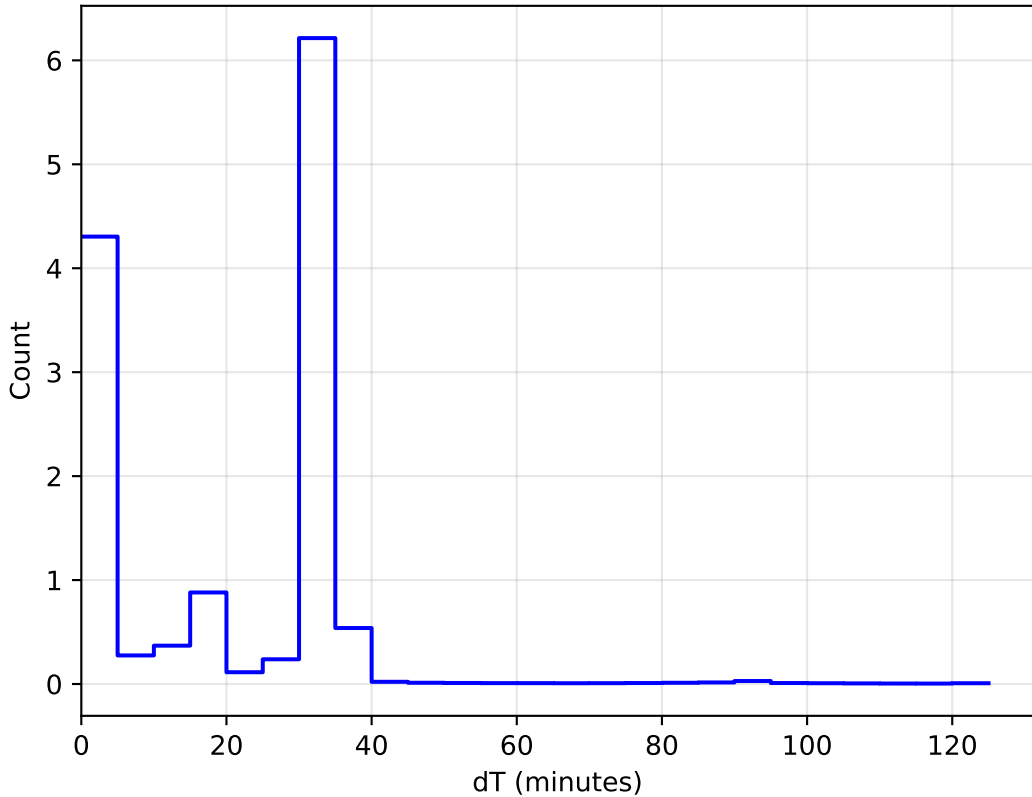
too_elab_2yr_r64_d3_ugrizy_v3.4_10yrs All sky: DeltaT Histogram 1e6
