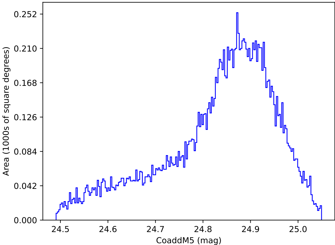
too_elab_2yr_r64_d3_ugrizy_v3.4_10yrs WFD y band: CoaddM5
