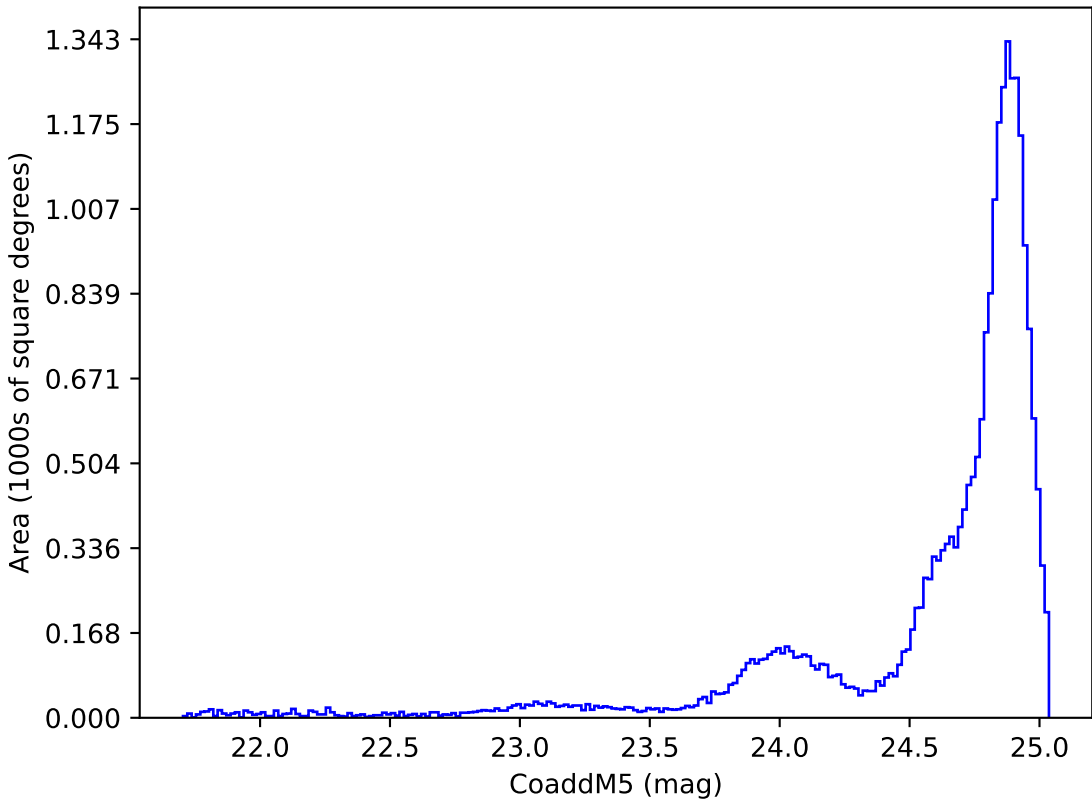
too_elab_2yr_r64_d3_ugrizy_v3.4_10yrs All sky y band: CoaddM5
