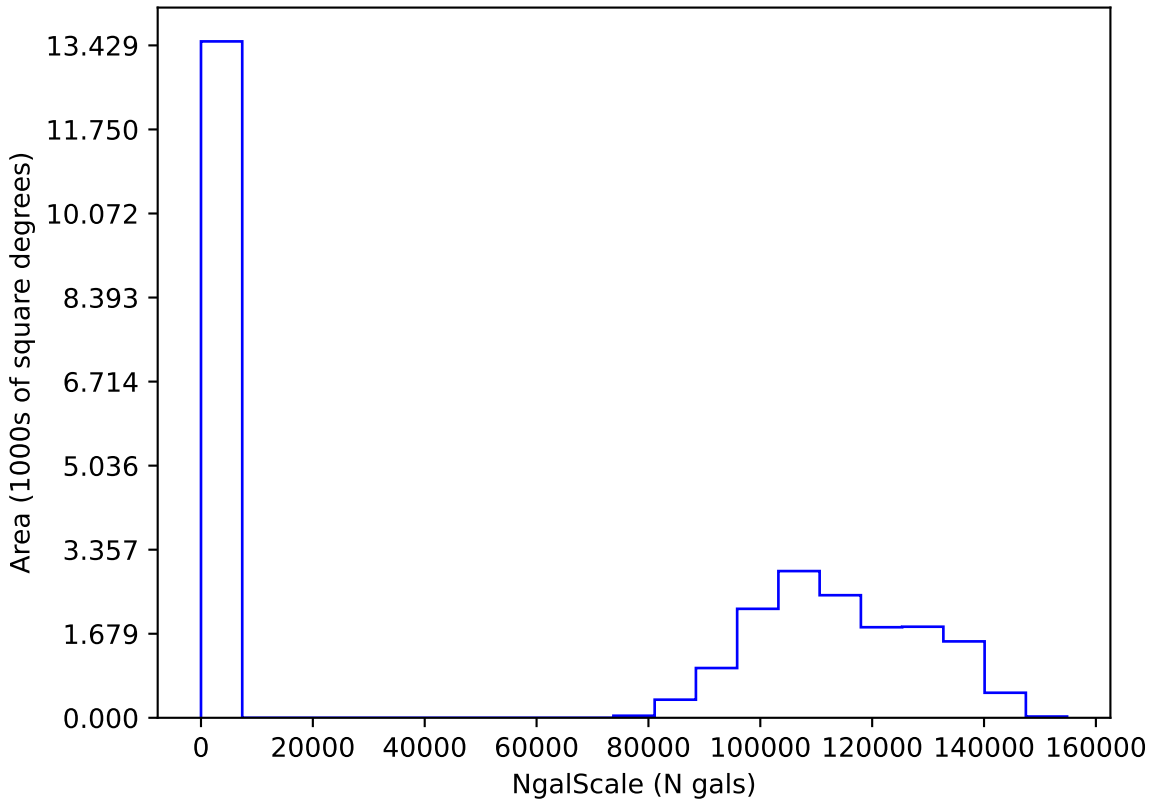
too_elab_2yr_r64_d2_ugrizy_v3.4_10yrs i: NgalScale
