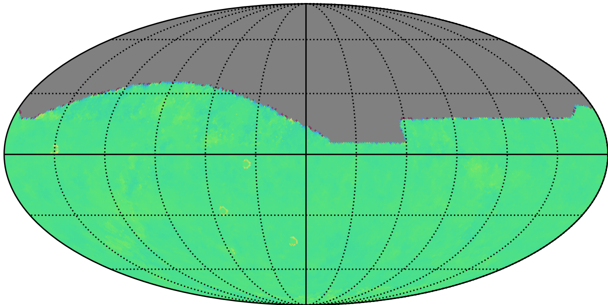
too_elab_2yr_r64_d2_ugrizy_v3.4_10yrs z: Kuiper rotTelPos
