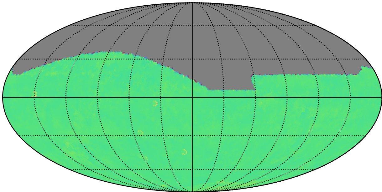
too_elab_2yr_r64_d2_ugrizy_v3.4_10yrs i: Kuiper rotTelPos
