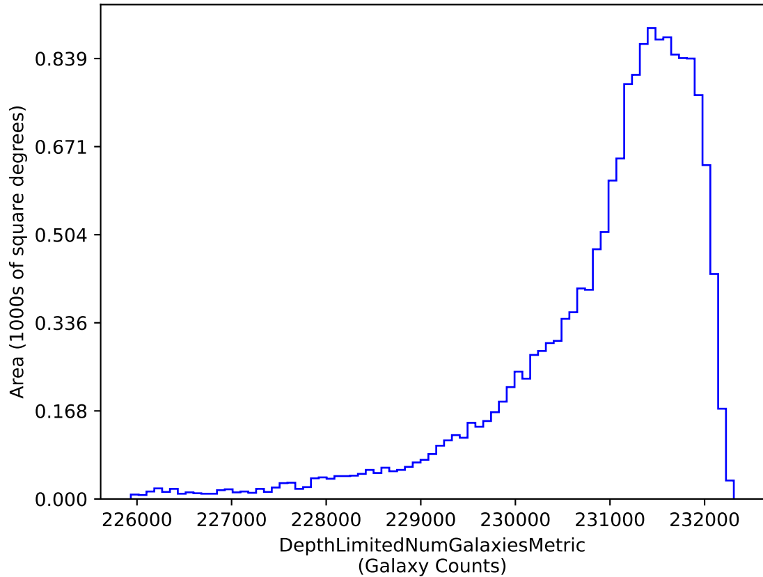
too_elab_2yr_r64_d2_ugrizy_v3.4_10yrs i band galaxies non-DD: DepthLimitedNumGalaxiesMetric
