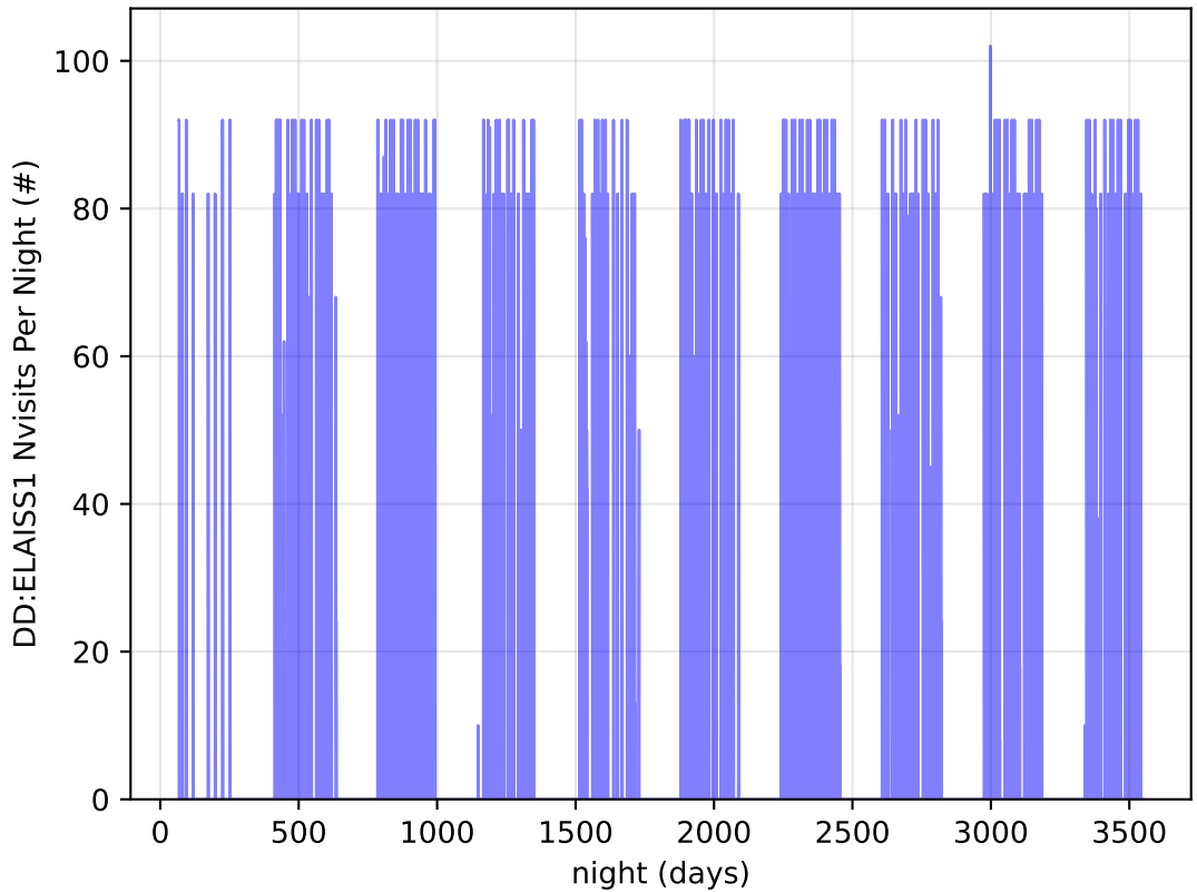
too_elab_2yr_r64_d2_ugrizy_v3.4_10yrs all bands: DD:ELAISS1 Nvisits Per Night
