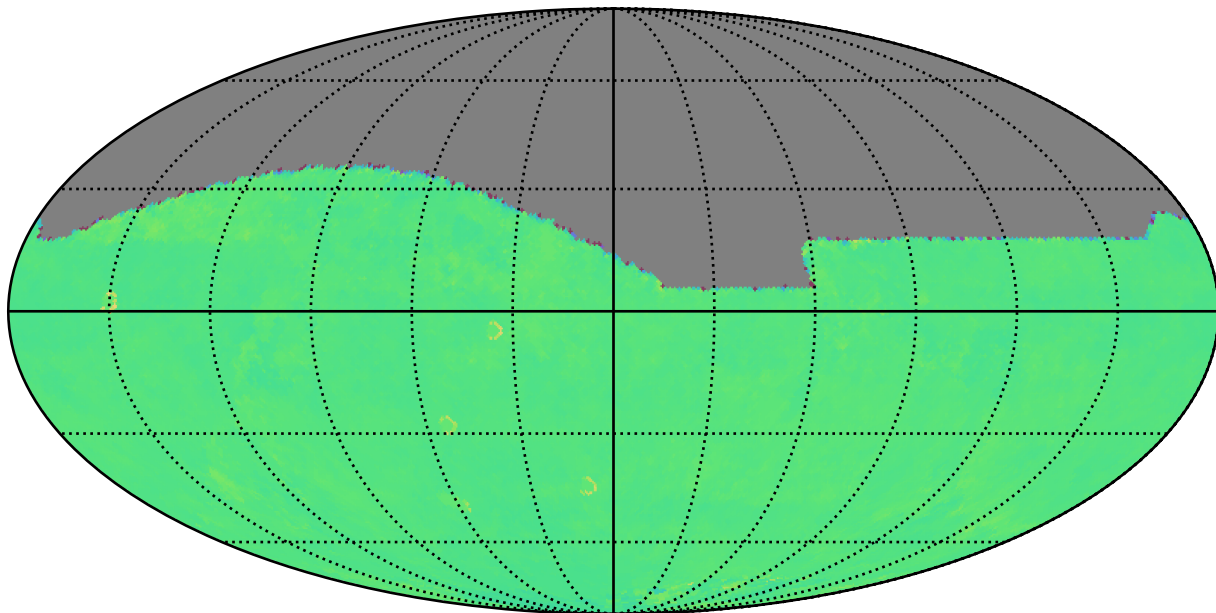
too_elab_2yr_r32_d3_ugrizy_v3.4_10yrs r: Kuiper rotTelPos
