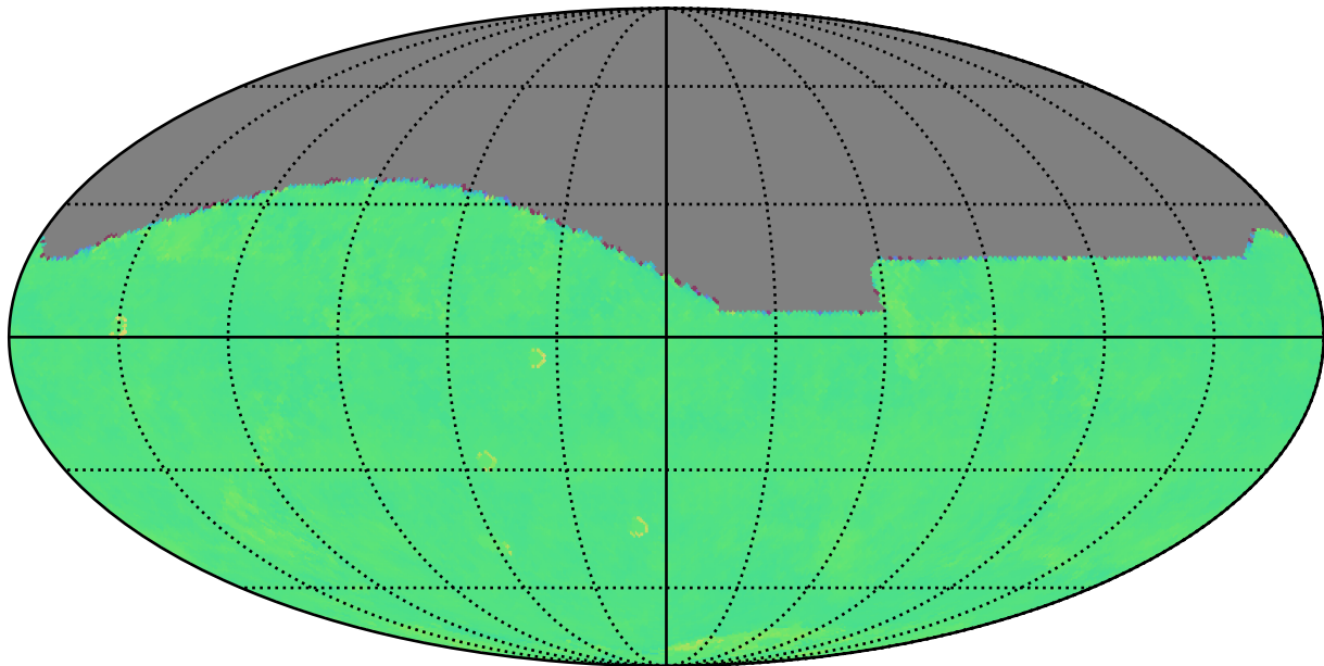
too_elab_2yr_r32_d3_ugrizy_v3.4_10yrs i: Kuiper rotTelPos
