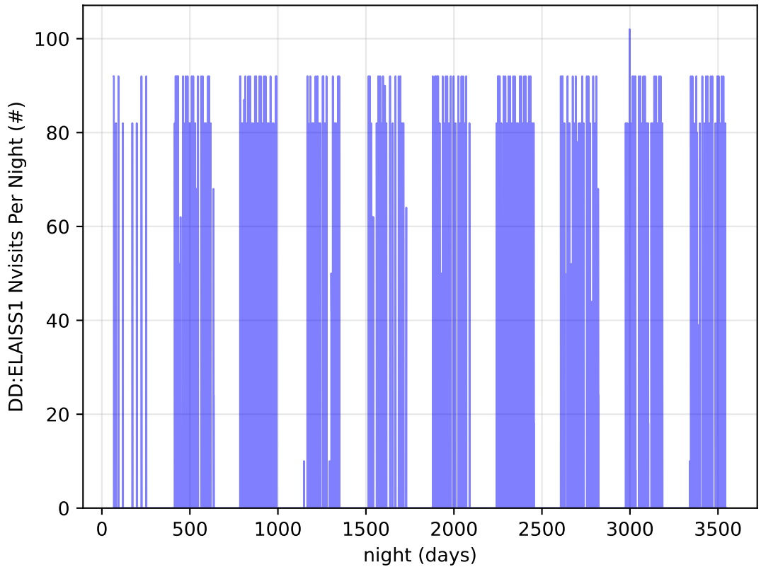
too_elab_2yr_r32_d3_ugrizy_v3.4_10yrs all bands: DD:ELAISS1 Nvisits Per Night
