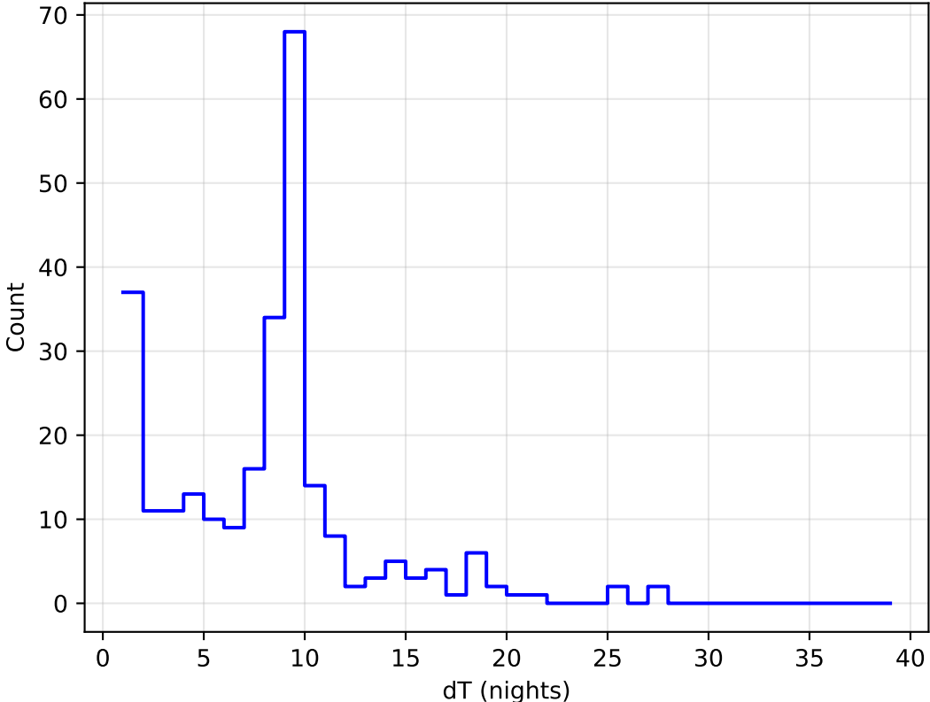
too_elab_2yr_r32_d3_ugrizy_v3.4_10yrs all bands: DD:ELAISS1 Delta Nights Histogram
