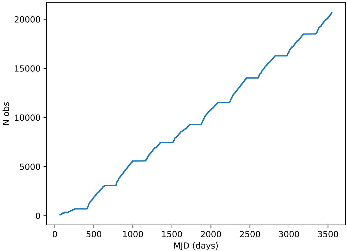
too_elab_2yr_r32_d3_ugrizy_v3.4_10yrs all bands: DD:ELAISS1 Cumulative NVisits
